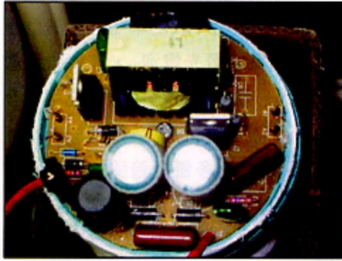
圖 2 省電燈泡燈帽內的電子式安定器
