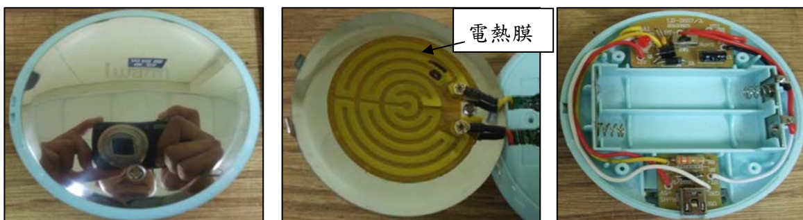
圖 3 採用鎳鎘電池及鹼性電池的電暖蛋；不具充電電路；發熱體:電熱膜 (購自樣品拆解)
