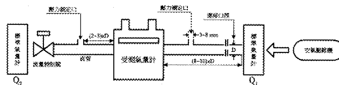
圖 B.2 氣量計測試配置參考圖例
